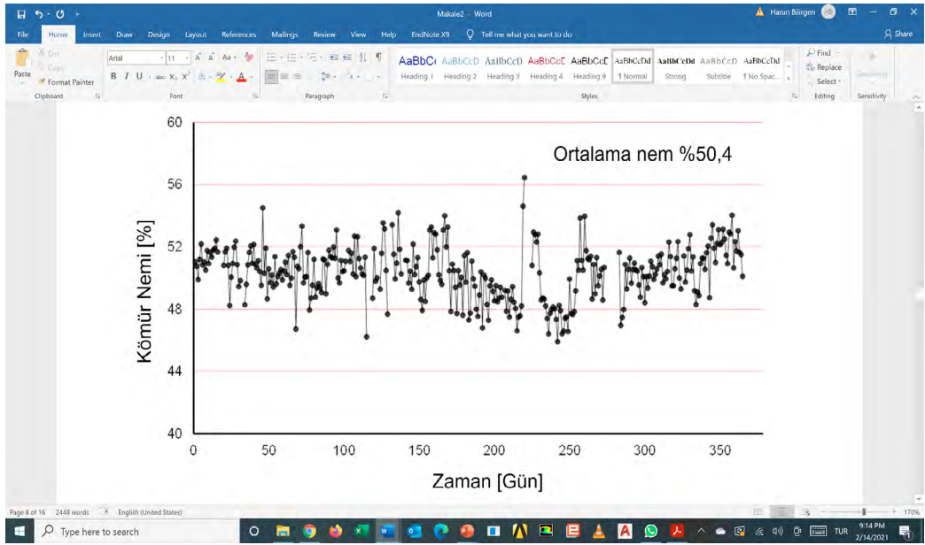
Şekil 12. Yerli Linyit Yakan Bir Termik Santralde Kömür Neminin Zamana Göre Değişimi
