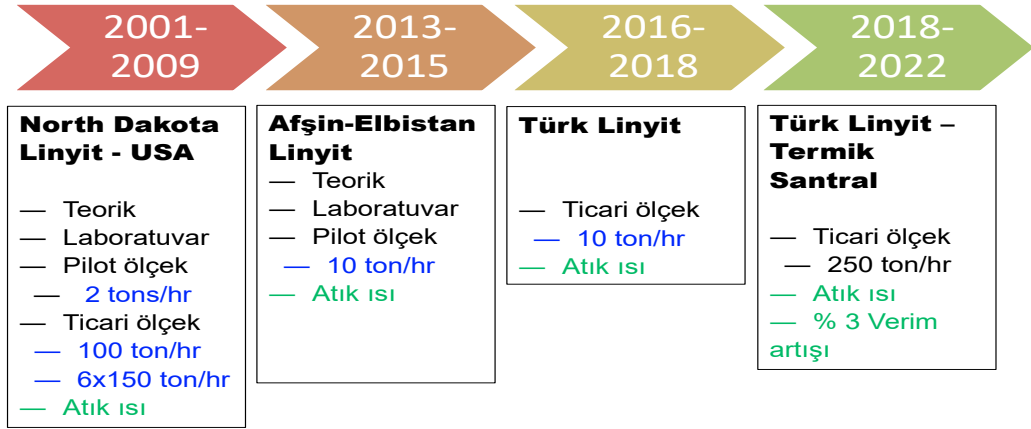
Şekil 10. Termik Santrallerdeki Atık Isı Kömür Zenginleştirme Teknolojisinin Kronolojik Gelişimi (Bilirgen, 2018)
