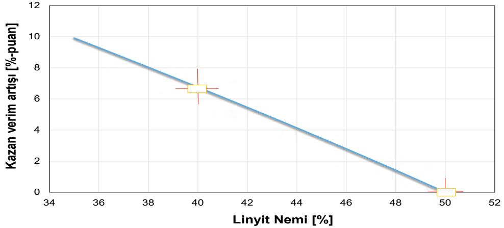
Şekil 14. Linyit Nemi ile Kazan Verimi Arasındaki İlişki
