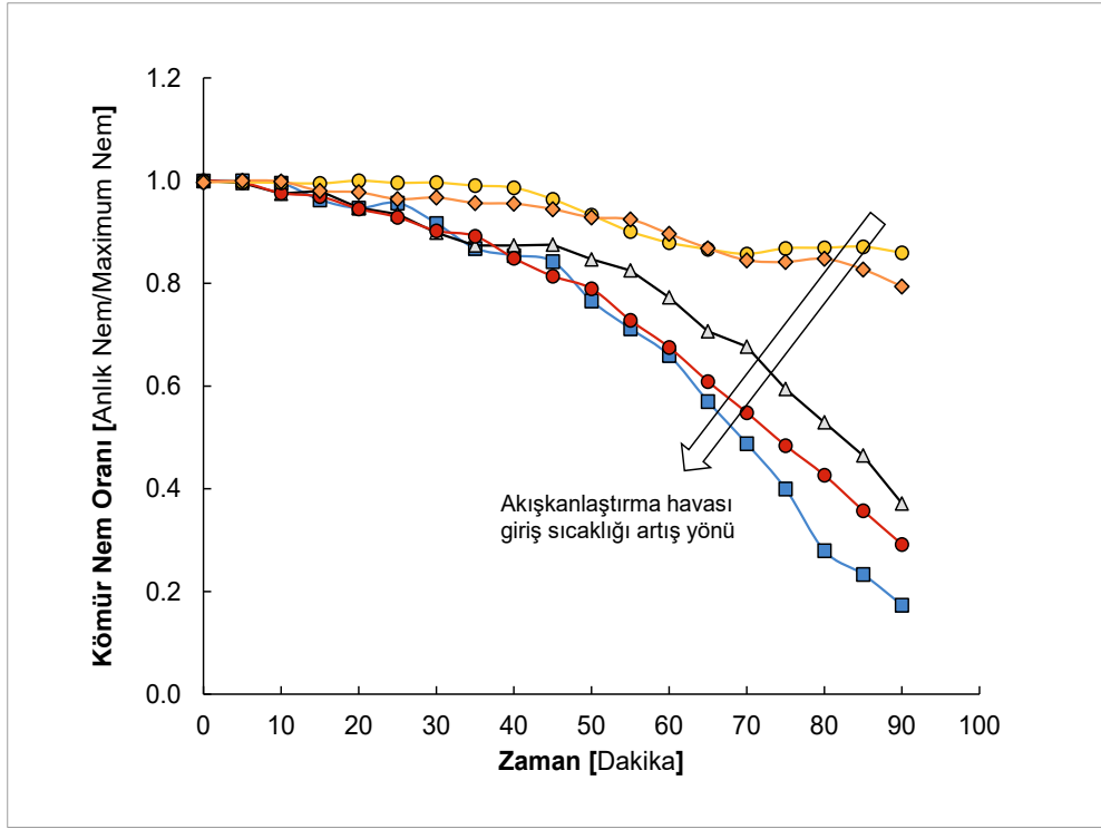
Şekil 6: Akışkanlaştırma Havası Sıcaklığına Bağlı Olarak Afşin-Elbistan Kömürü Kuruma Karakteristiği
