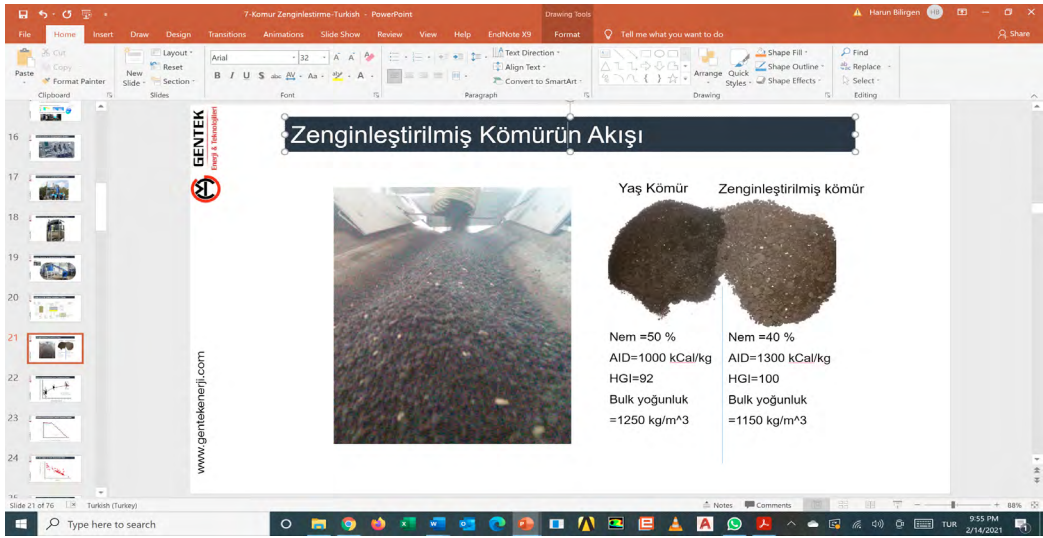
Şekil 11. Pilot Ölçekli Kömür Kurutma ve Zenginleştirme Sistemi – Afşin-Elbistan A Termik Santrali
