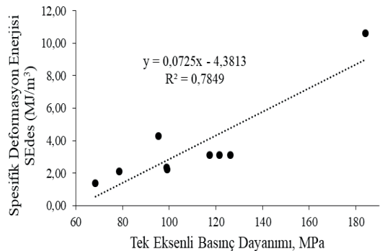
Şekil 9. Spesifik deformasyon enerjisi ile tek eksenli basınç dayanımı arasındaki ilişki
