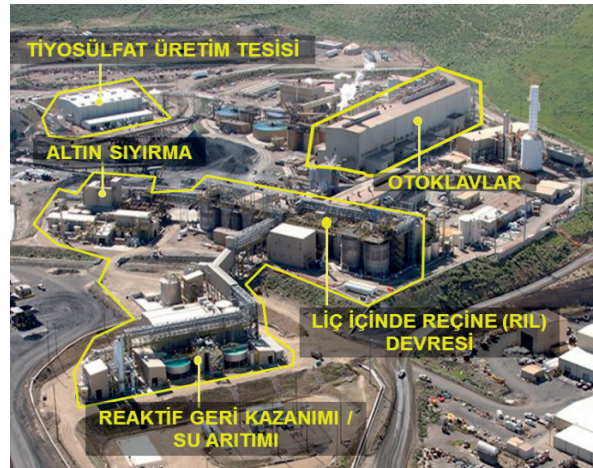
Şekil 7. Barrick Gold Şirketine ait Goldstrike tiyosülfat liçi tesisi (Nevada, ABD) (Barrick Gold, 2016; Choi, 2016)
