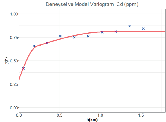
Şekil 2. Cd (ppm) özneliğinin deneysel ve model variogramı
