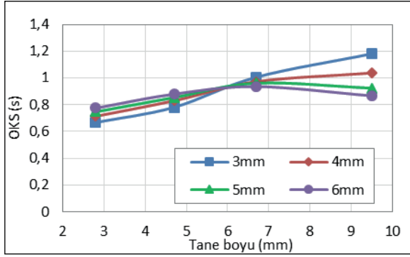
Şekil 7. Tanelerin farklı titreşim genliklerindeki ortalama kalma süreleri
