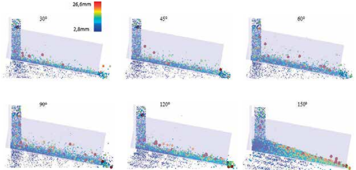
Şekil 15. Farklı titreşim yönlerinde yapılan simülasyonlarda, sistemin dengeye ulaşmasının ardından elde edilen ekran görüntüleri
