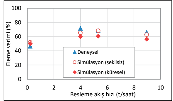
Şekil 7. Çeşitli besleme akış hızlarında gerçekleştirilen pilot test ve simülasyonların eleme verimliliği
