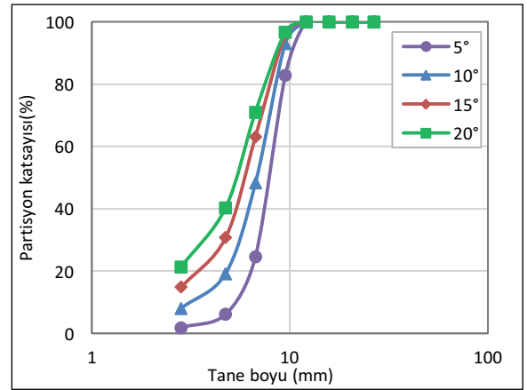
Şekil 3. Farklı elek eğimlerinde elde edilen partiyon eğrileri
