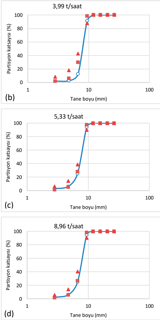
Şekil 8. Çeşitli besleme hızlarında yapılan pilot testler ve simülasyonların partiyon eğrileri
