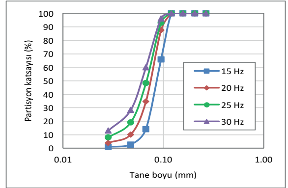
Şekil 9. Farklı titreşim sıklıklarında elde edilen partisyon eğrileri
