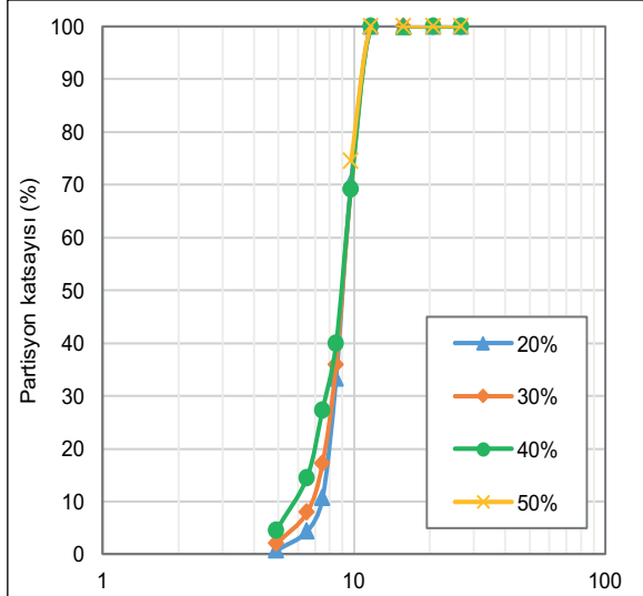
Şekil 21. Farklı miktarda yakın boyutlu malzeme içeren beslemeler için partisyon eğrileri
