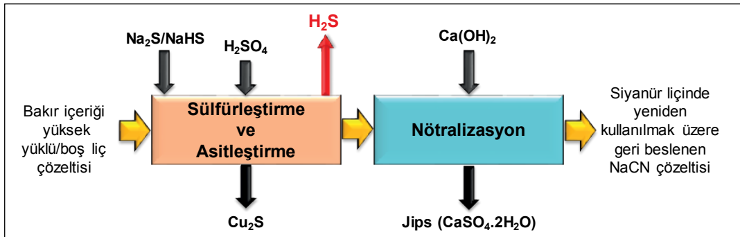
Şekil 5. SART prosenin şematik akım şeması (Nodwell vd. (2012)'den değiştirilerek)
