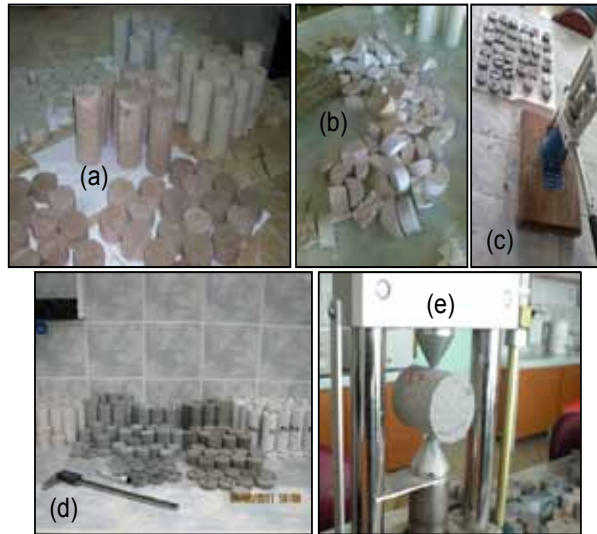
Şekil 1. Biyomikritik kireçtaşları (a) ve eksenel deney sonrası örnekler (b ve c), diğer kayaç gruplarından bazıları (d) ve çapsal deneyin uygulandığı (e)
