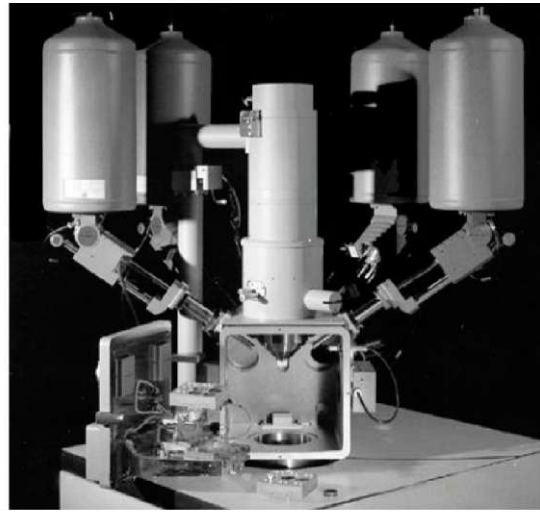
Şekil 5. QEM*SCAN sistemi
